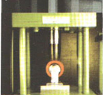
회전 시험 / Revolving test
